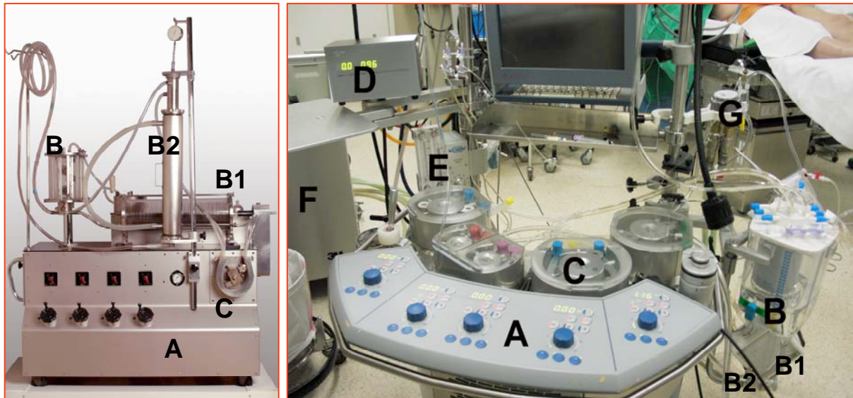
Figure 7.2 : Machines de CEC. A gauche: machine historique de Livio-Mettraux, Lausanne 1962. A droite: machine actuelle. A: console centrale avec commandes des pompes (boutons bleus). B: réservoir veineux. B1: oxygénateur. B2 : échangeur thermique (couplé à l'oxygénateur et au réservoir dans la machine moderne). C: pompes. D: écrans de contrôle. E: Mélangeur de gaz et vaporisateur. F: bac fournissant de l'eau à température variable pour l'échangeur thermique. G: circuit de cardioplégie. A 50 ans d'écart, les pompes n'ont pas changé, mais l'oxygénateur s'est complètement transformé.
